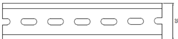
ADMISSIBLE DIN-RAIL: TS35/7.5 OR TS35/15
